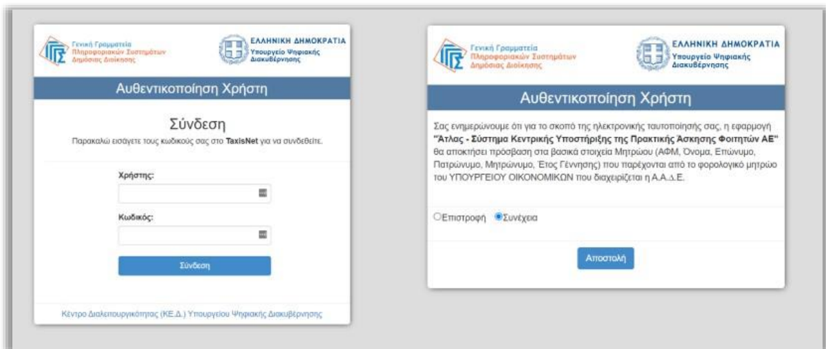
Εικόνα 3.2 - Σελίδα TaxisNet
